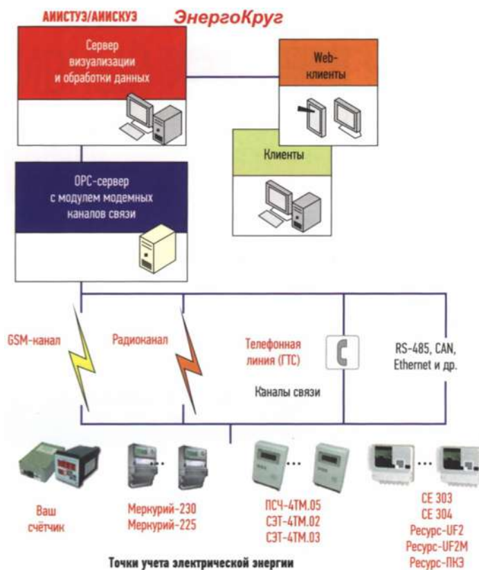
РИС. 3. ► Архитектура автоматизированной системы учета электроэнергии
