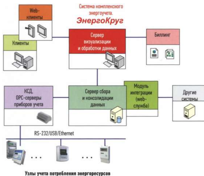
РИС. 2. ► Архитектура АСКУЭ
